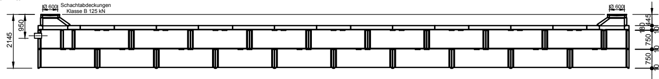
Längsschnitt
