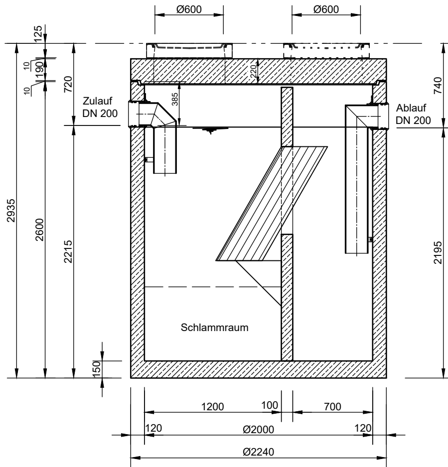
Schnitt A-A
