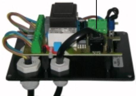
Steckbuchse
