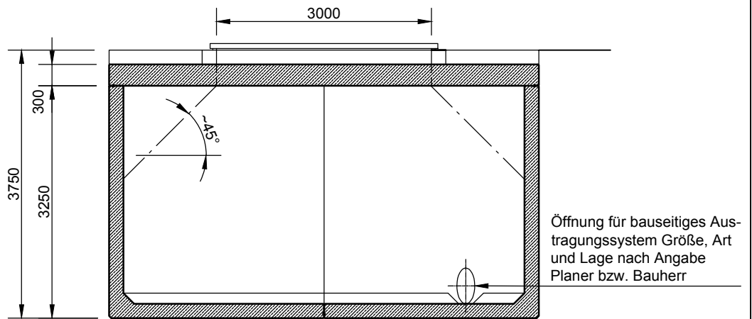
Schnitt B-B
