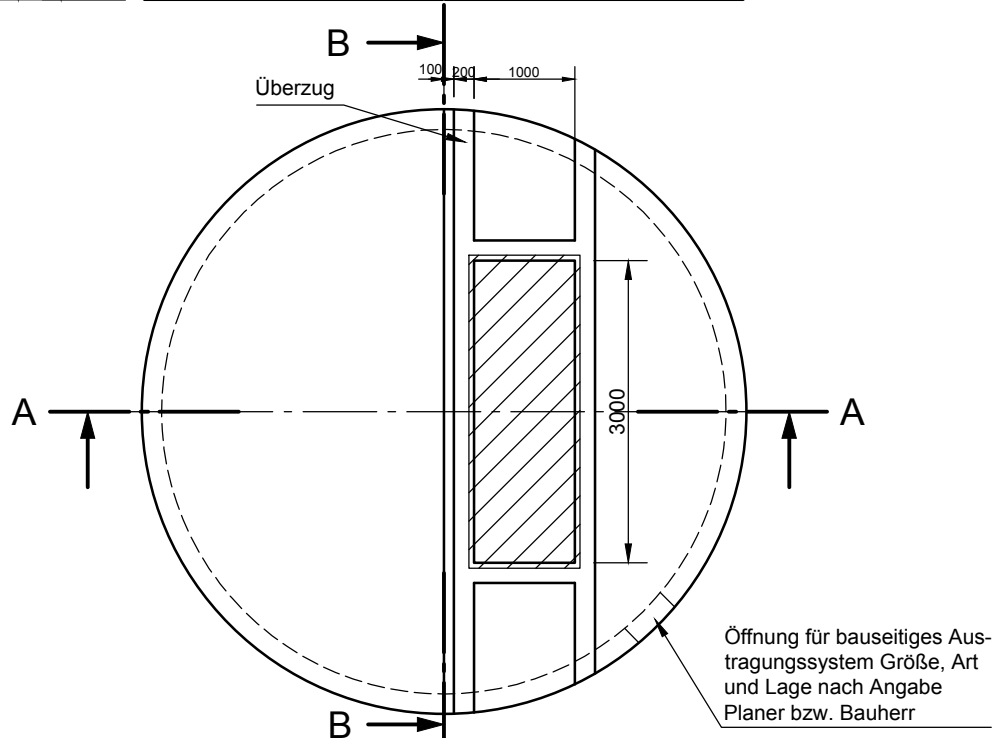
Grundriss
