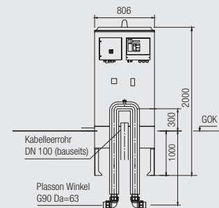
Rückstauschleife LevaStop
