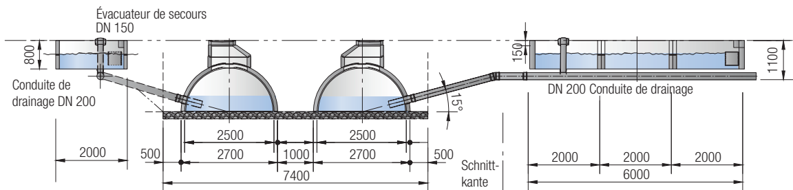
Installation d'infiltration Innodrain
